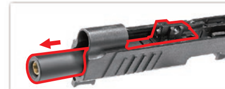
Retire el cañón.
