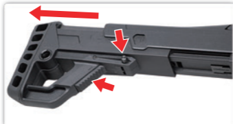
壓下解除鈕及調整鈕拔除後托。
