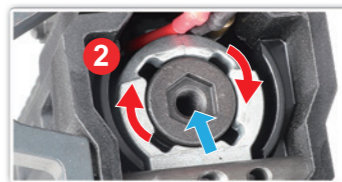
使用內六角(8mm)內壓尾頂桿之後轉動至開口處。
