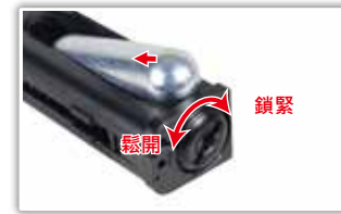
使用六角板手工具鬆開CO2氣瓶旋蓋，放入CO2氣瓶，再鎖緊旋蓋並裝回彈匣底座。
