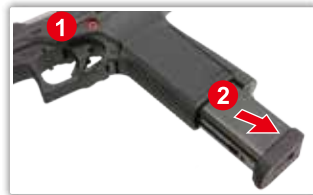
1. Abaisser l'arrêtoir chargeur. 2. Retirer le chargeur.
