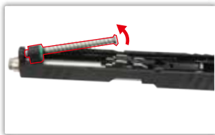
向前推擠覆進程後向上移出。
