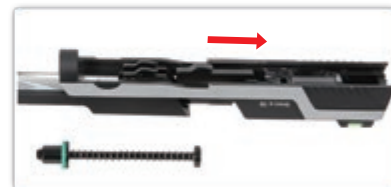
將滑套向後推出。
