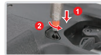
Empuje hacia abajo el tornillo con el destornillador de , luego gire 90 grados en sentido antihorario.
