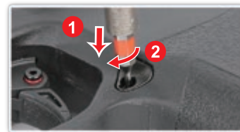
使用一字起子將彈匣釋放鈕壓下並順時針旋轉90度旋緊螺絲。
