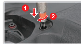
Utilisez un tournevis à tête plate, et tournez de 90 degrés dans le sens horaire pour verrouiller.
