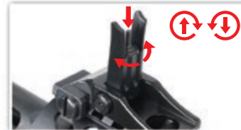
Presione el boton para ajustar la mira arriba o abajo.
