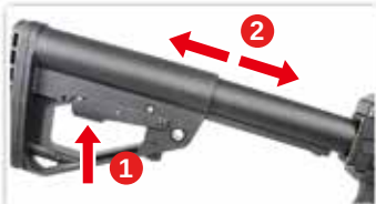
1. 壓下調整片。 2. 調整適合之槍拖長度（可6段調整）。
