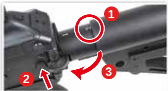
1. 將槍托調整至第二段。 2. 按下折疊托釋放鈕。 3. 將托桿向槍身左側折疊。
