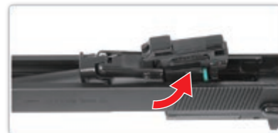
取出外管。 分解後可進行適度清潔及噴塗砂油保養。
