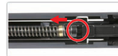
Poussez le guide de ressort vers l'avant et compressez le ressort.
