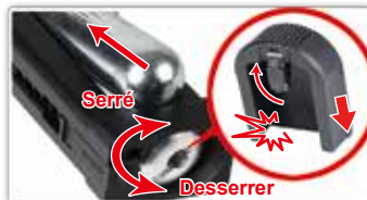
Serré Desserrer Sortez la clé hexagonale du talon et utilisez-la pour desserrer le bac à cartouche en bas du chargeur. Insérez la cartouche de CO2 dans le chargeur et resserrez.
